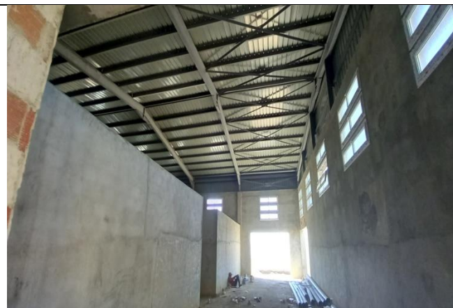
أشغال تركيب السقف الحديدي
