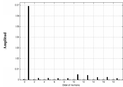
Structure N°04 : THD=13,48%
