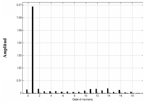
Structure N°02 : THD=12,03%
