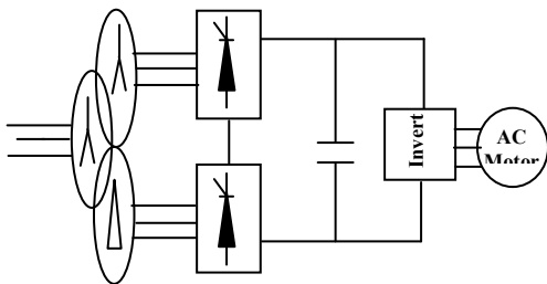
Fig. 2 Twelve pulse rectifier
